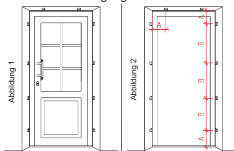
Bild 5 Befestigungsabstände
