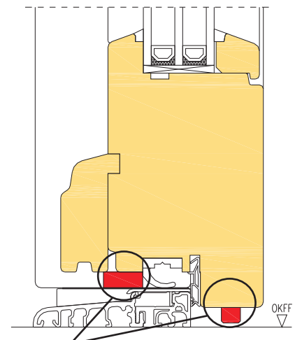
Sicherung und Scheuerschutz
